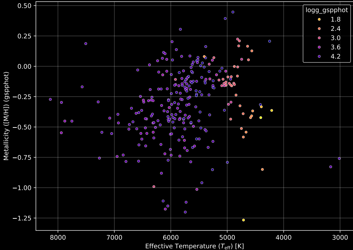
GALAH DR4 Field: [7171] Stellar Population Parameters (n= 265)
