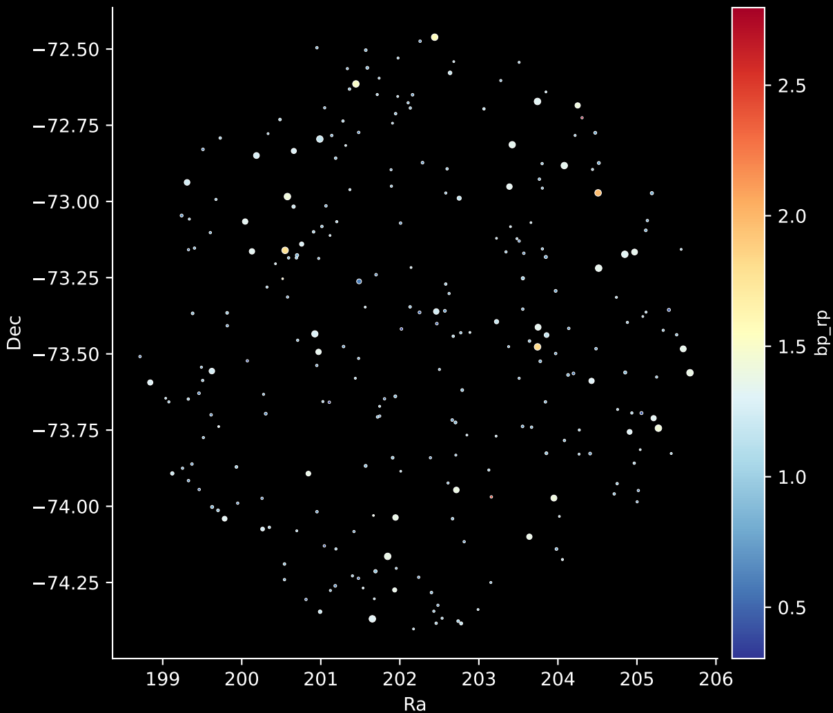
GALAH DR4 Field: [7171] Stars: 265
