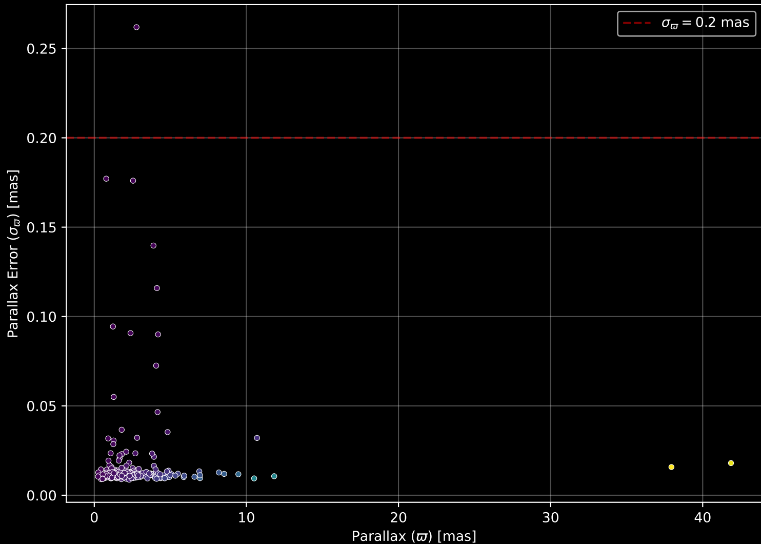
GALAH DR4 Field: [7171] Parallax Quality (n= 265)
