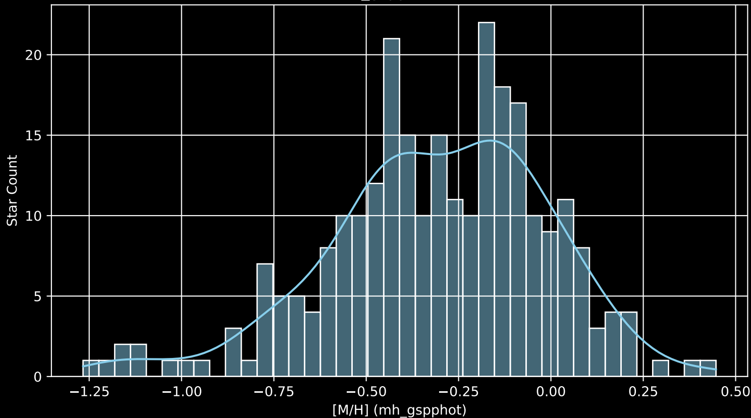
GALAH DR4 Field: [7171] [M/H] (mh_gspphot) (n= 265)
