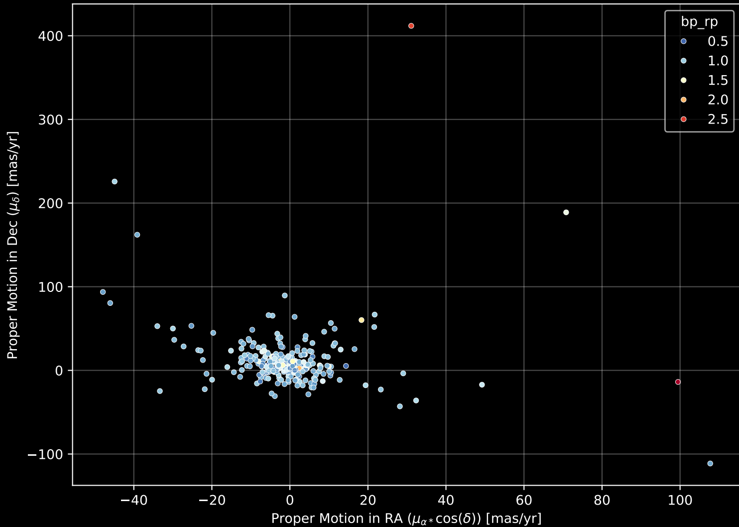
GALAH DR4 Field: [7171] Proper Motion Diagram (n= 265)
